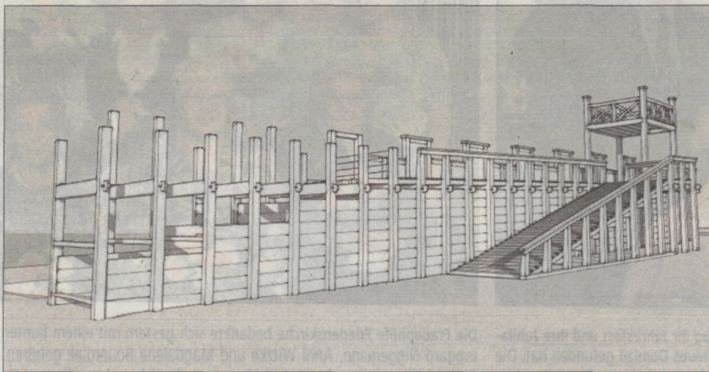
So soll die Holz-Erde-Mauer aus Blickrichtung Westen aussehen: Wie in römischer Zeit führt eine Rampe auf die Mauer. Am unfertigen westlichen Ende (l.) können Besucher Schritt für Schritt verfolgen, wie die Befestigung konstruiert ist. ▪ Animation: Dr. Peterse
